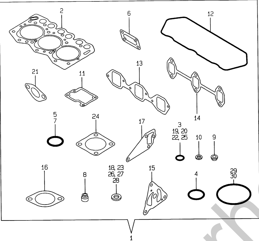
Fia.17.GASKET SET 17.GASKET SET
